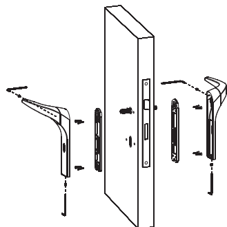
MONTAŻ KLAMKI MODEL 2055
