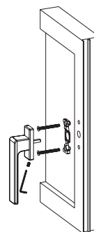
MONTAŻ KLAMKI OKIENNEJ I BALKONOWEJ
