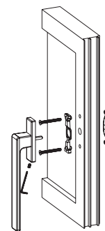
MONTAŻ KLAMKI OKIENNEJ I BALKONOWEJ
